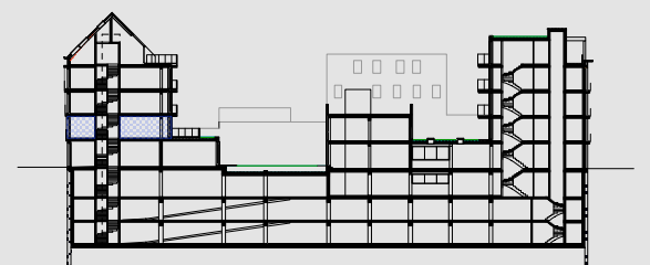
SNEDE
