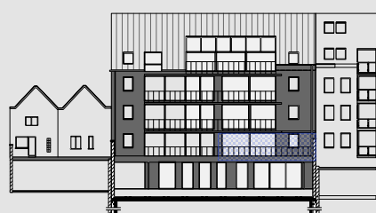
ACHTERGEVEL
